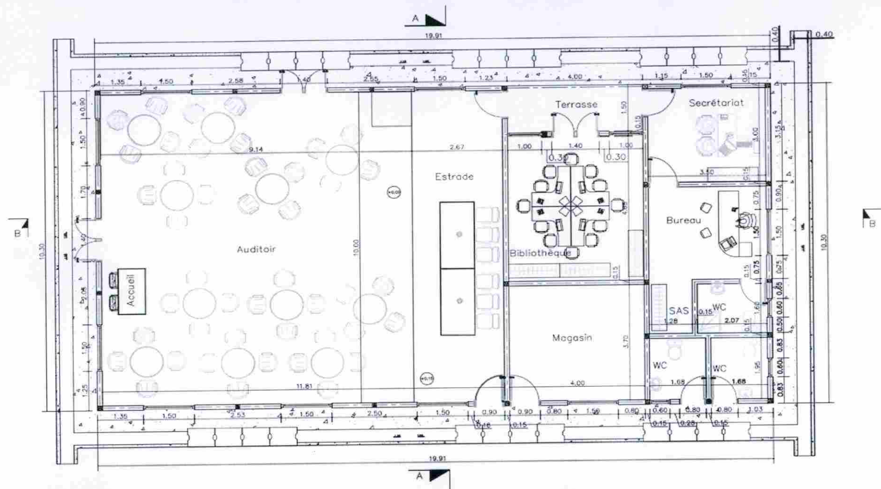
PLAN DE DISTRIBUTION CASE COMMUNAUTAIRE E:1/50
